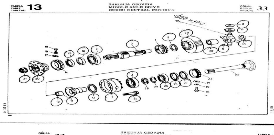
Diferencijal srednje osovine FAP 2626 BK (krst diferencijala \phi 22\text{mm} \times 150\text{mm} )
